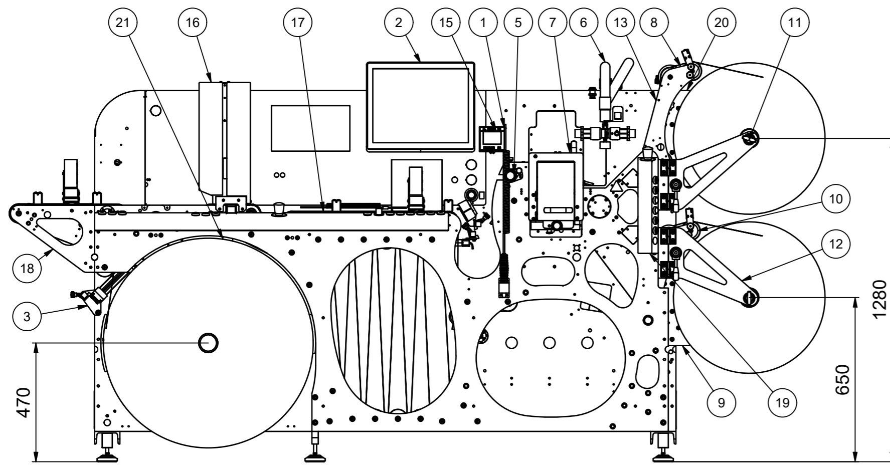
A-A ( 1 : 15 )
